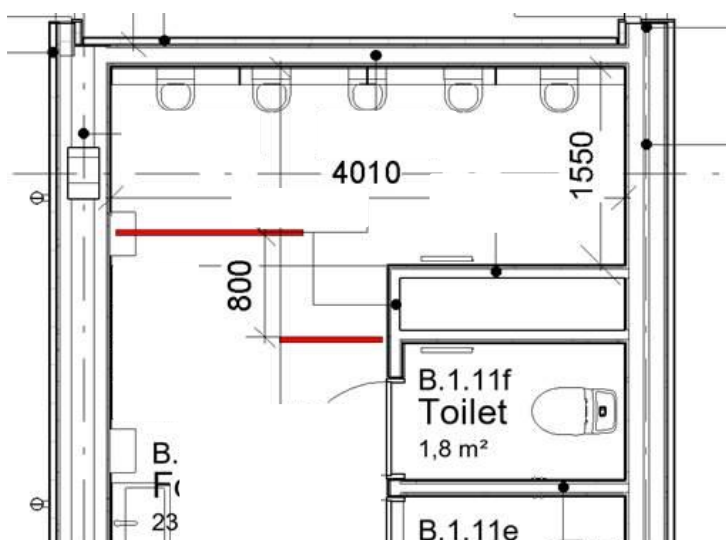
Løsning 1 Fælles toilet med urinaler - udsnit
