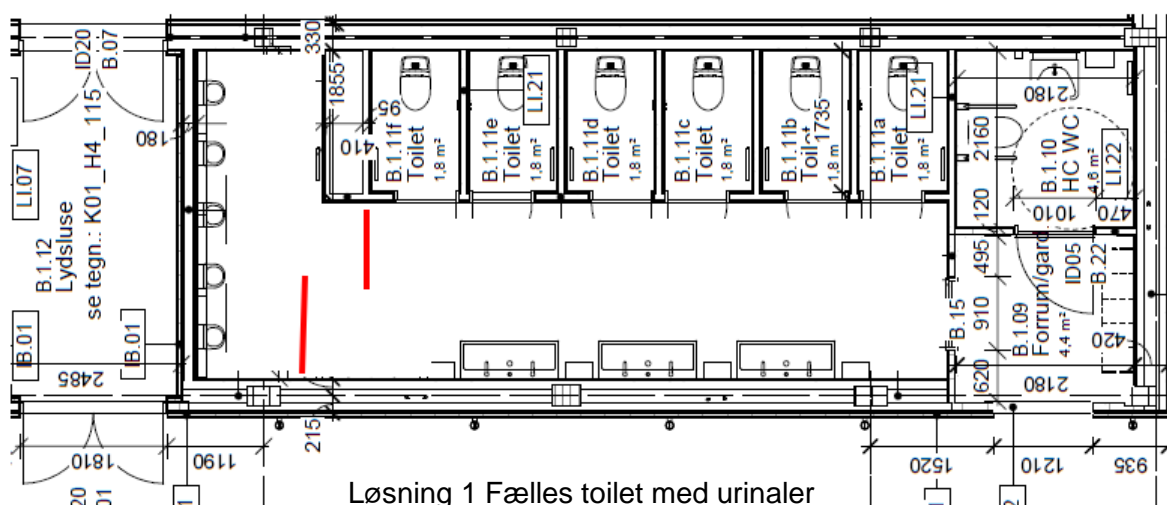
Løsning 1 Fælles toilet med urinaler - udsnit
